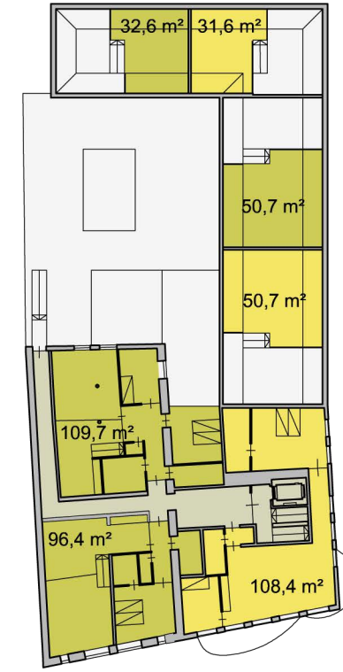
3e verdieping 3 woningen
